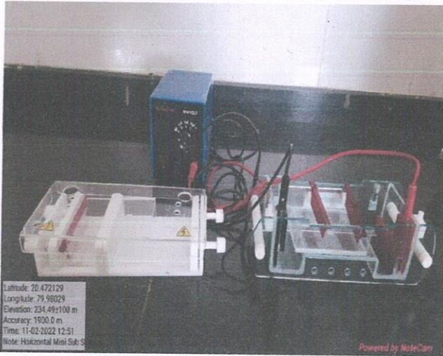
HORIZONTAL MINI SUB SYSTEM
